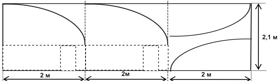
Схема раскроя листа сотового поликарбоната (6×2,1 м) для покрытия торцов теплицы
